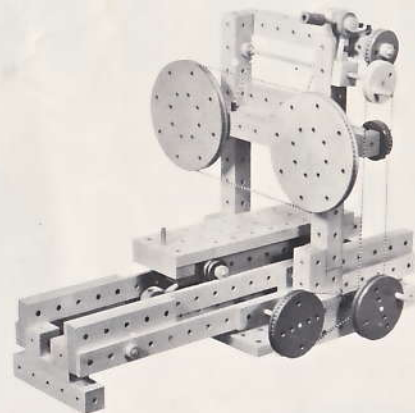
Horizontal-Bandsäge aus Matador Nr. 4
