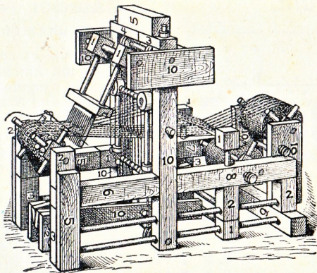
Webstuhl aus Matador Nr. 4. Damit kann man tatsächlich Bänder weben.
