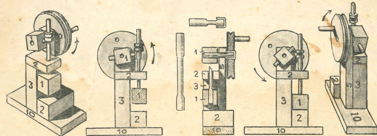
244. Dochwerk. Stamping-mill. Bocard. Macchina da tritare il minerale. Molino de quebrantar. Tlukárna (Stoupa). Tłuczakarnia rud. Młyn stępowy. Zuzó mŭ. Kölyümalom. Pukværk (Stampe). Stampmolen.
